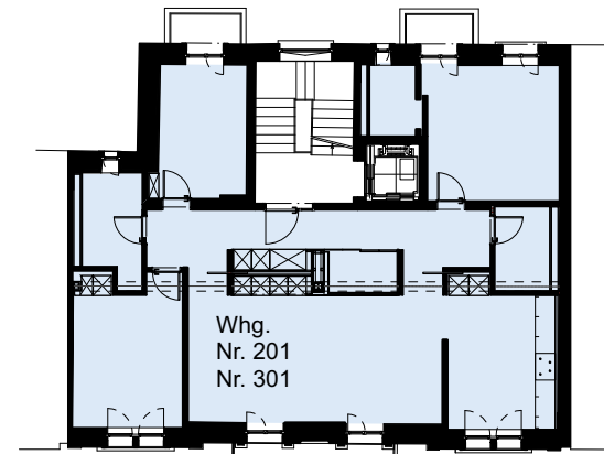
2./3.Obergeschoss
